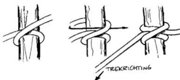
Mastworp (eindknoop)
