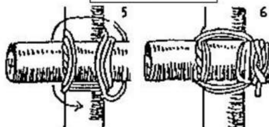
Kruissjorring
