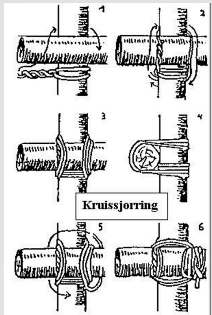
Kruissjorring
