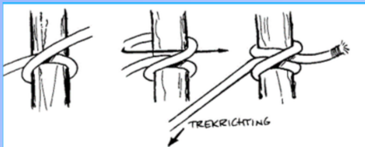
Mastworp (eindknoop van een sjorring)
